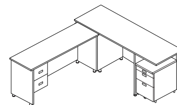
COD-100 (1800×900×720)
