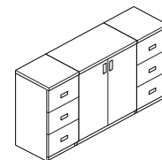
BC-160 (1800×480×735)
