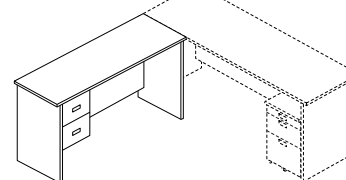
BD-102 (1260×480×670)
